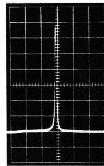
Abb. 1 e. N_p = 80 mW, Leistungsverstärkung 32 dB, \sqrt{G} B = 21,5 MHz (Empfindlich- keit des Empfängers um 13 dB verringert).
