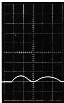
Abb. 1 a. Pumpleistung N_p = 0 , Resonator bei para- magnetischer Reso- nanz angepaßt.
