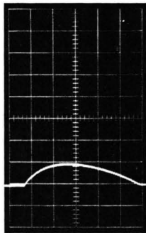
Abb. 1 b. Resonatorverluste bei N_p > 0 ausgeglichen, der Resonator ist „transparent“.
